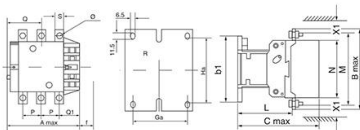
CJX2-D115~620
